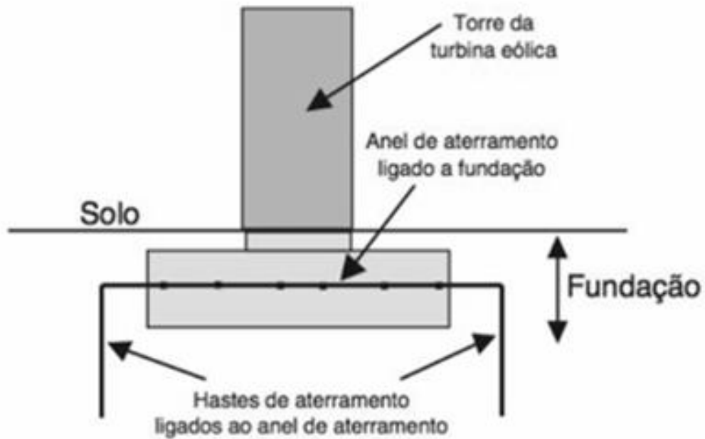
Figura 61. Aterramento
