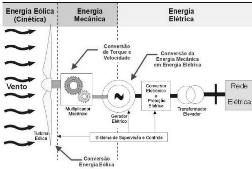
Figura 51. Funcionamento de um Aerogerador.
