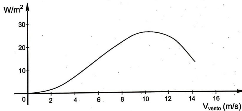
Figura 20. Distribuição da Potência.
