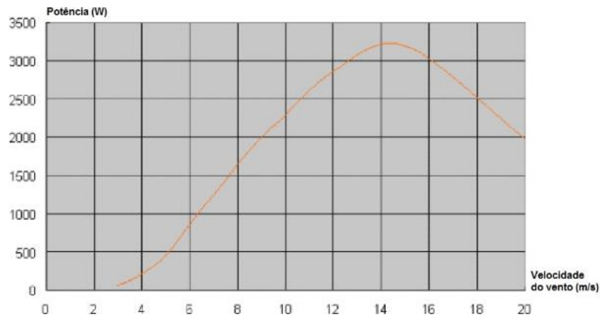
Figura 68. Curva de Potência do Modelo escolhido.
