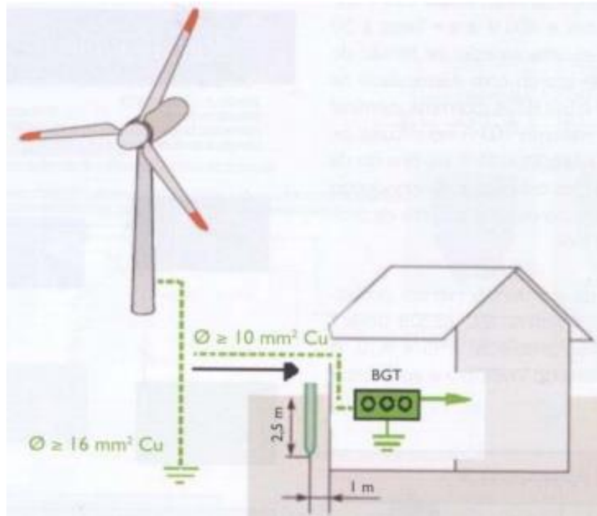
Figura 58. Esquema de Ligação Terra na Turbina Eólica.
