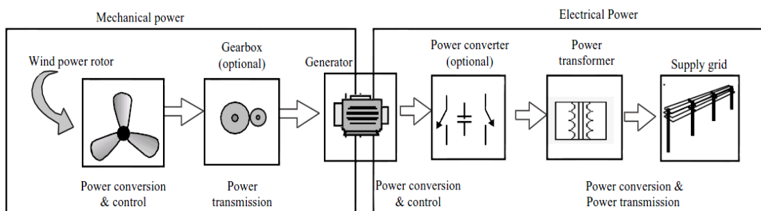
Figura 29. Principais Componentes para produção de Energia Eólica.
