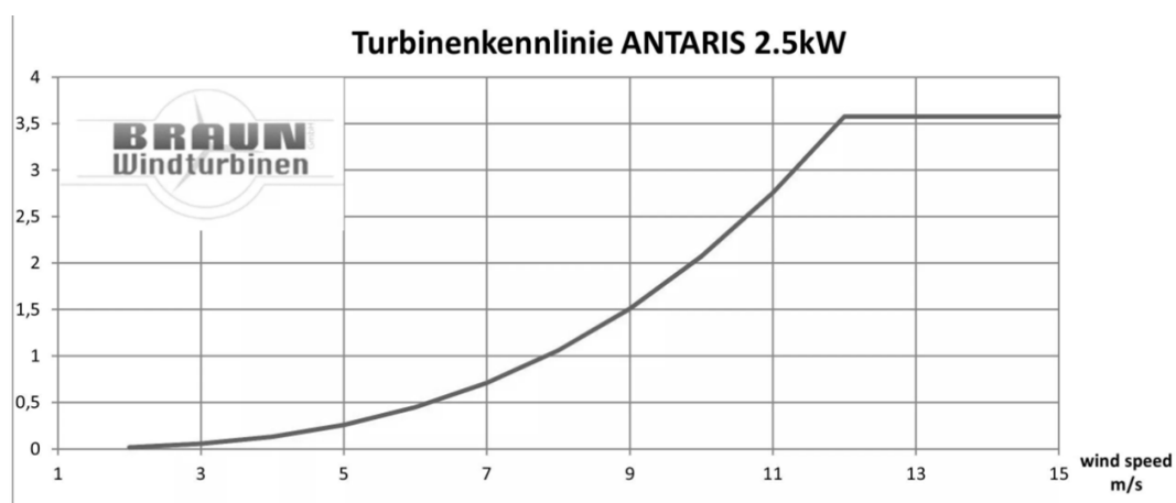
Figura 72. Curva de Potência ANTARIS 2.5 kW
