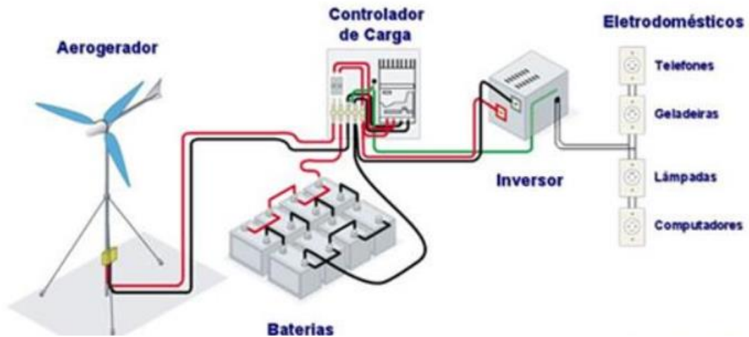
Figura 45. Sistema Isolado de Microgeração Eólica.
