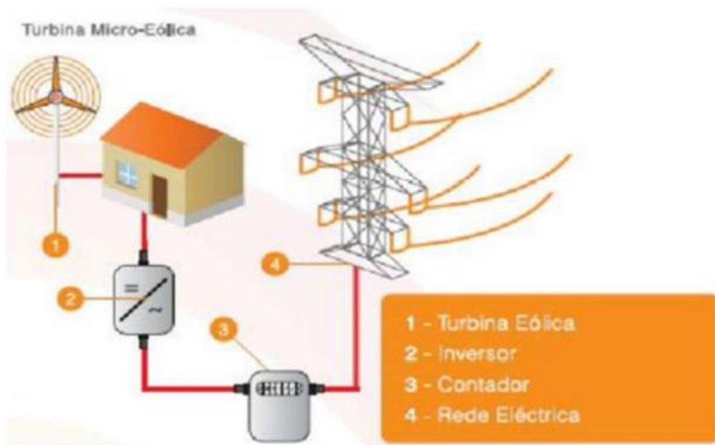
Figura 41. Demonstração de um Sistema Micro-eólico conectado à rede.
