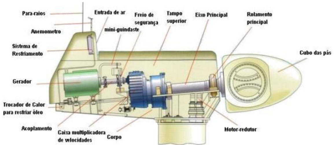
Figura 33. Componentes de uma Turbina Eólica de Eixo Horizontal.
