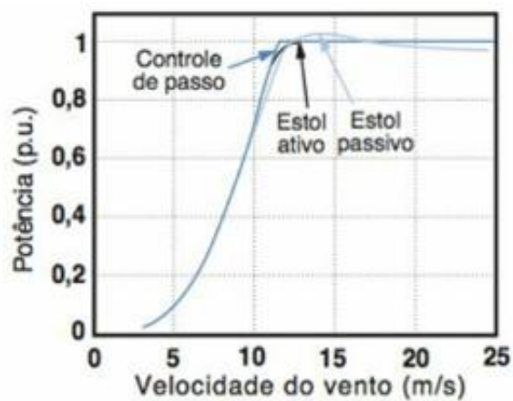
Figura 22. Características dos Tipos de Controle.
