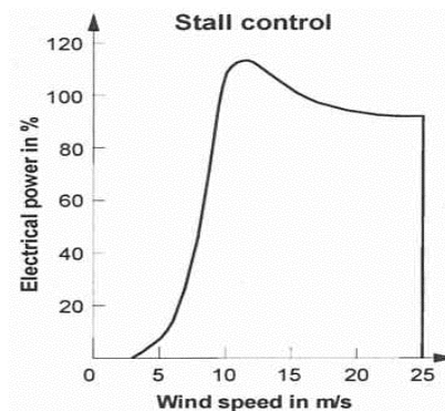
Figura 26. Curva de Controle Stall
