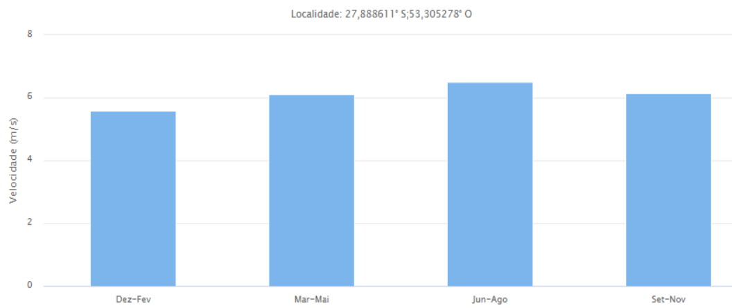
Figura 54. Velocidade média Sazonal de Vento a 50 m de altura [m/s]
