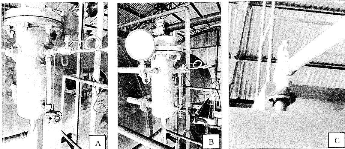
Figura 7A, 7B e 7C: Visor de nível d'água (A), manômetro de pressão e nível d'água (B), válvula de segurança (C)
